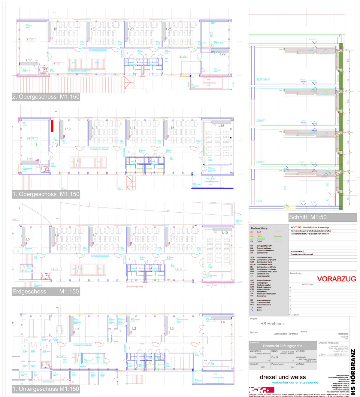
Obr. 17 a,b Ukázka projektové dokumentace decentrálního řešení základní škola Hörbranz (Drexel und Weiss)
