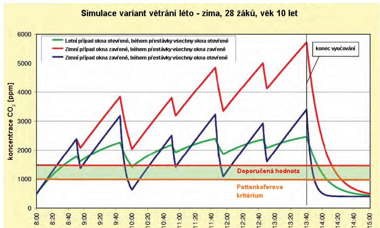
Obr. 6 Simulace přirozeného větrání učebny pro různé varianty větrání a jeho dopadu na koncentraci oxidu uhličitého. Výsledky simulace ukazují, že i v ideálních případech větrání pře přestávky nedochází k dostatečnému provětrání prostoru. (Měření kvality vzduchu v školách v Horním Rakousku, Amt der OÖ. LR., Abt. Umwelt- und Anlagentechnik)
