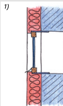
1) Osazení nového okna do poloviny tloušťky tepelné izolace (okno vysunuto na konzolách)
