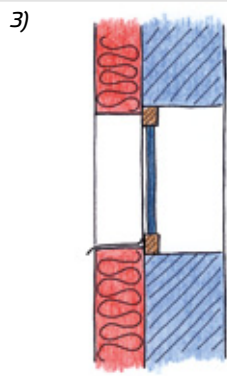
3) Osazení nového okna na líc nosného zdiva, tepelná izolace přesahuje přes rám okna
