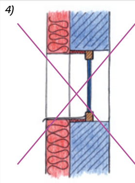
4) Osazení nového okna na místo původního; toto řešení volíme pouze ve výjimečných případech, pokud předchozí řešení nejsou použitelná
