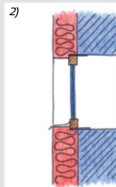
2) Osazení nového okna do tepelné izolace – zjednodušené řešení (okno též vysunuto na konzolách)
